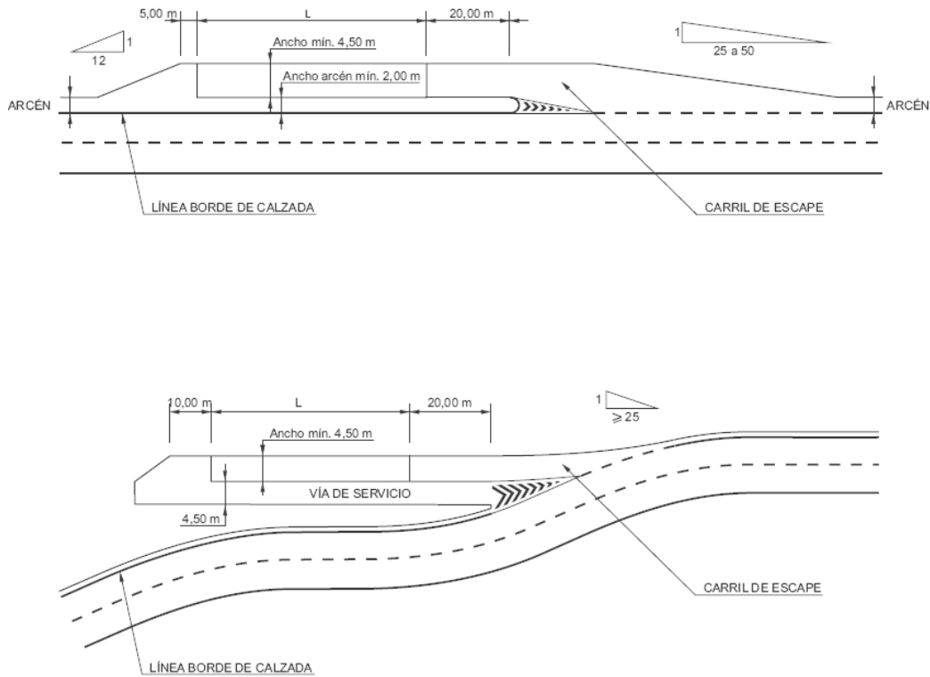
FIGURA 8.27. LECHOS DE FRENADO.
