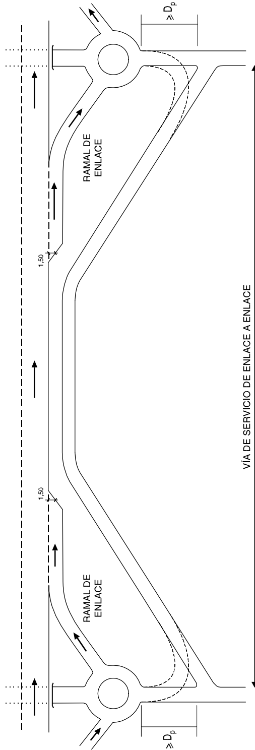
FIGURA 9.6. CONEXIÓN DE VÍAS DE SERVICIO A TRAVÉS DE ENLACES.
