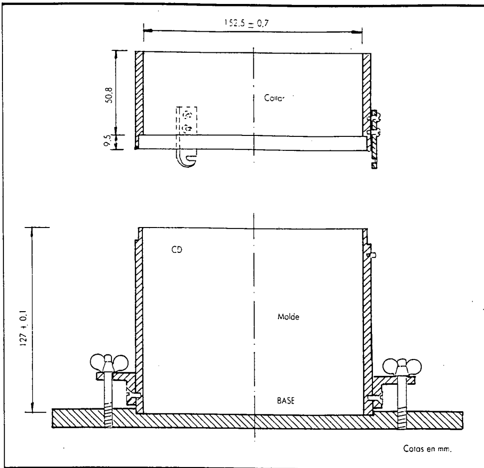
FIGURA 1. Molde Próctor modificado.
