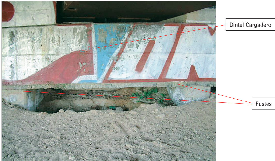
FIGURA 115. CARGADERO SOBRE FUSTES.
