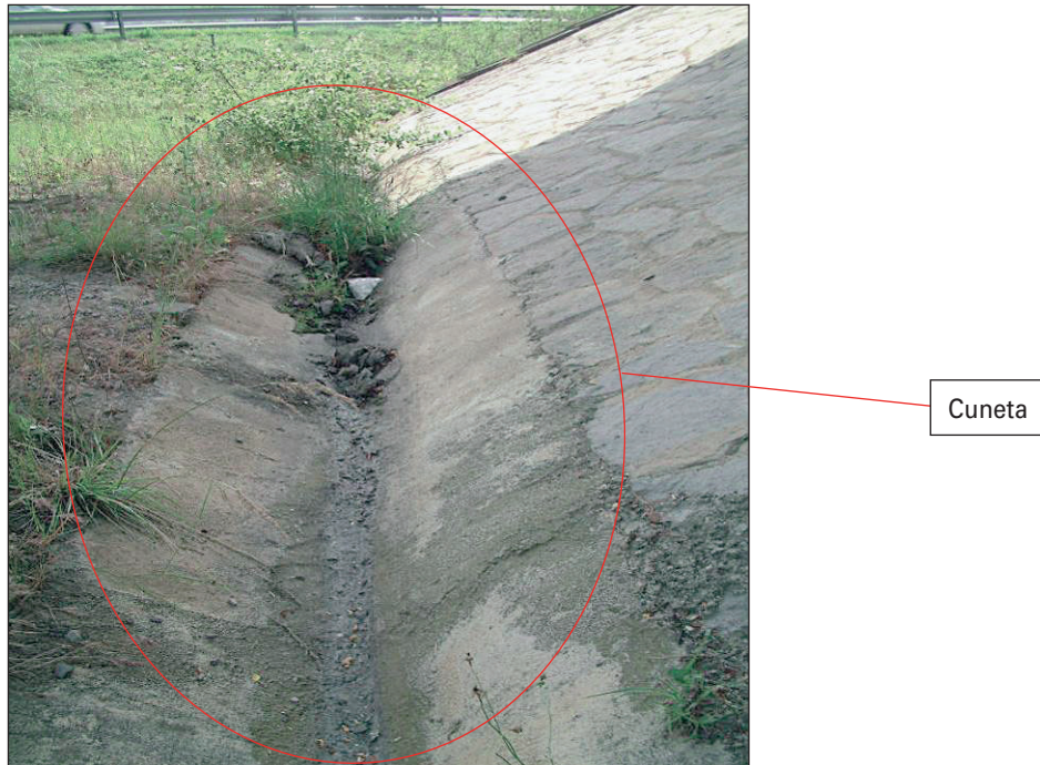
FIGURA 157. PROTECCIÓN DEL TERRAPLÉN MEDIANTE CUNETAS.
