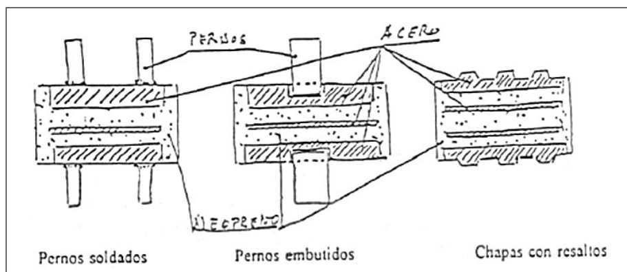
FIGURA 86. APOYO ANCLADO.
