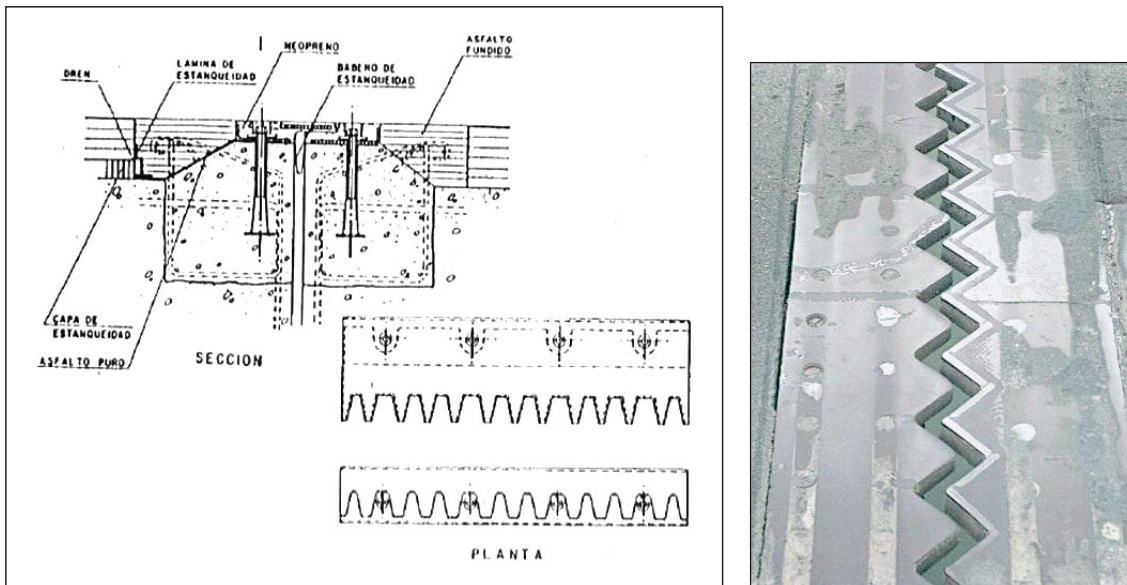
FIGURAS 136 Y 137. JUNTA DE TIPO «PEINE».
